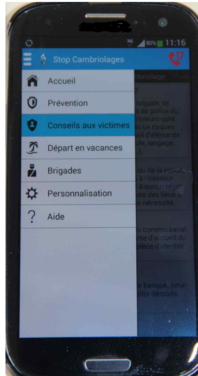
Menu déroulant
