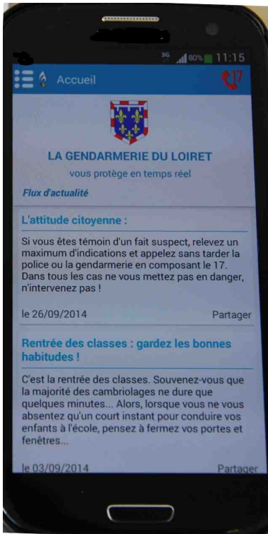
Page d'accueil
